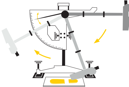
Pendulum Test
